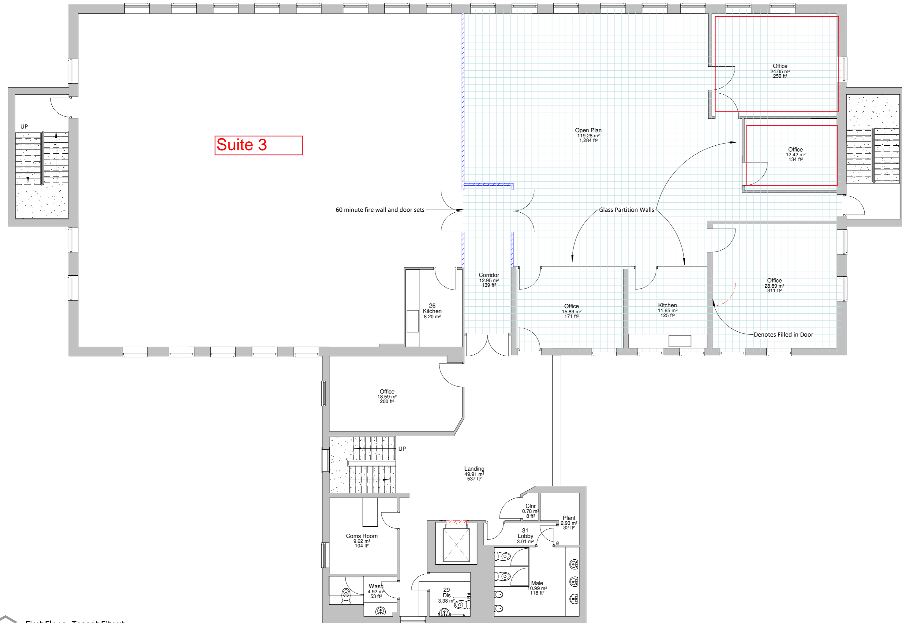
1 First Floor - Tenant Fitout 1:100
